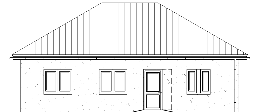
Vorderansicht
