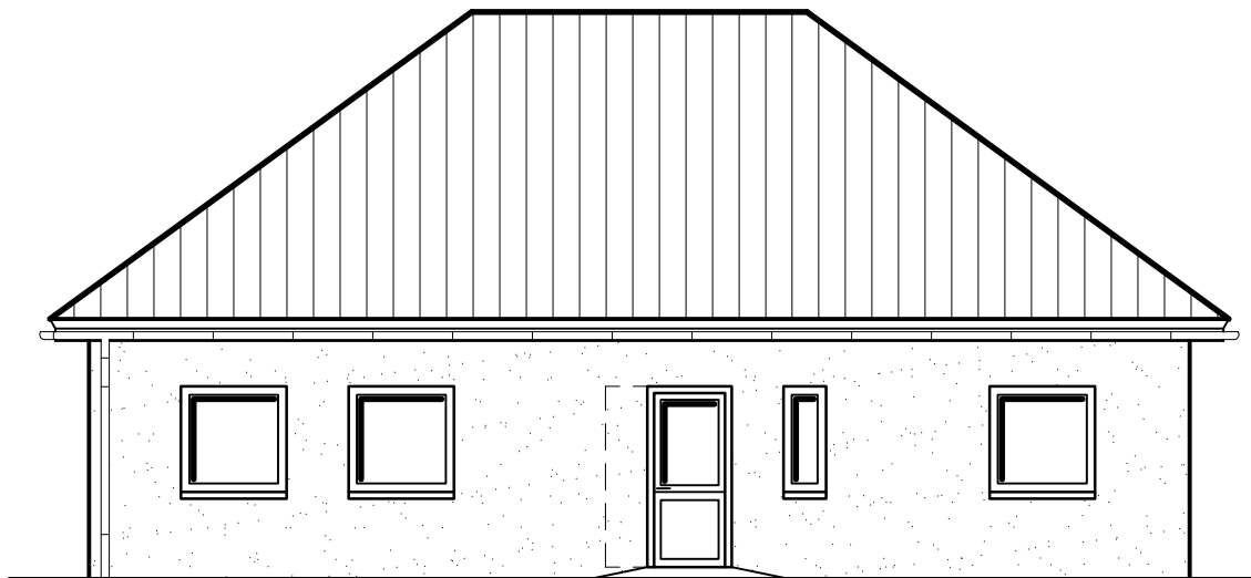
Vorderansicht
