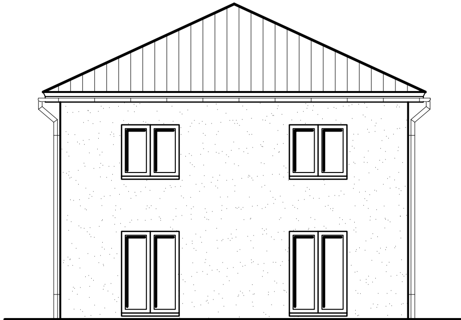
Rückansicht
