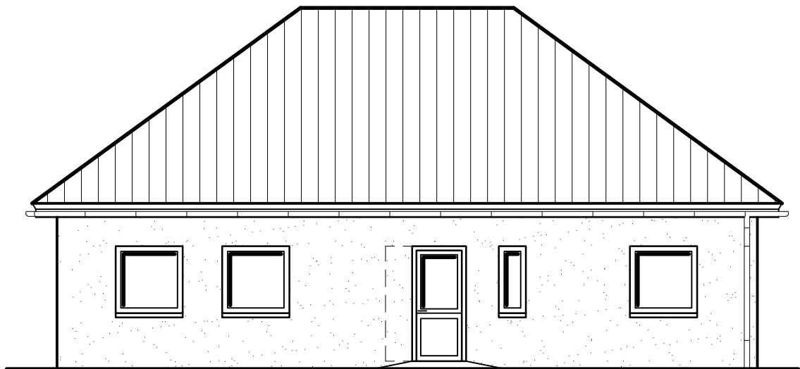
Vorderansicht
