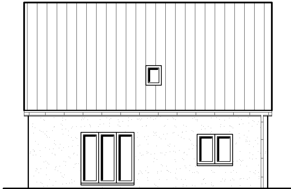
Rückansicht
